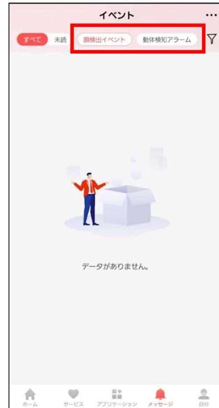
Android OS
